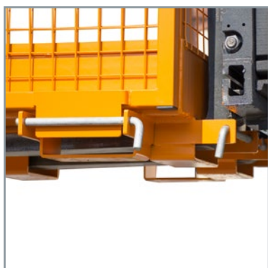
↑ Die Sicherungsbolzen schützen vor unbeabsichtigtem Abrutschen.
